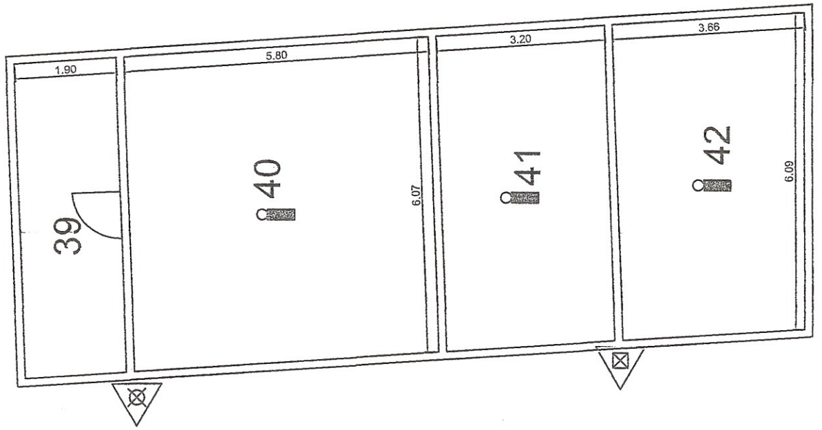
PLANTA BAIXA - GARAGEM
